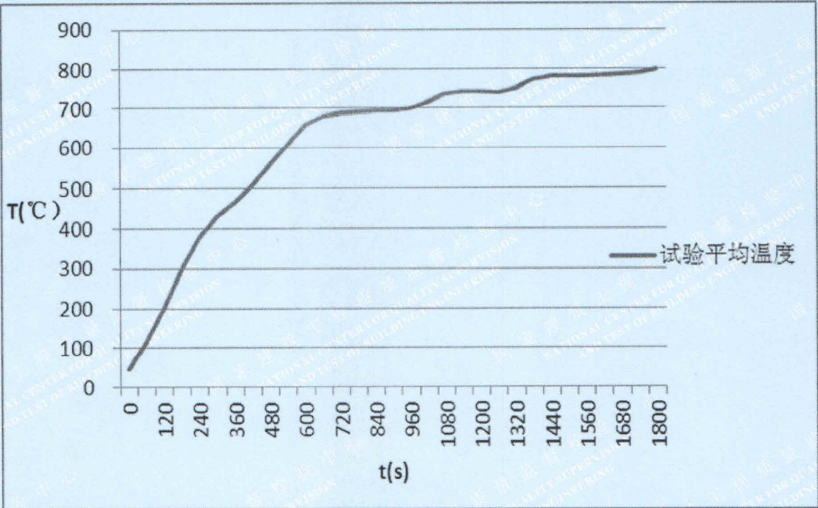
图 1 试验温度记录曲线图
