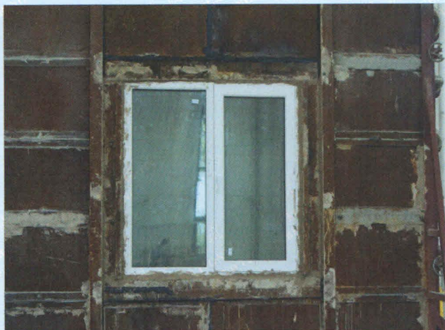
图2 耐火完整性试验前样品状态图
