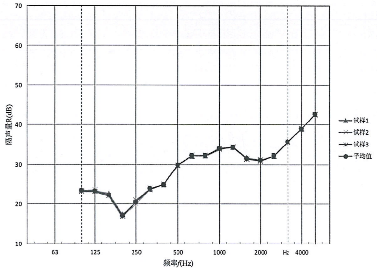
图1 空气声隔声性能检测结果曲线图
