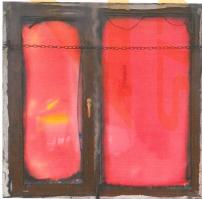
照片二 耐火试验结束时试件情况
