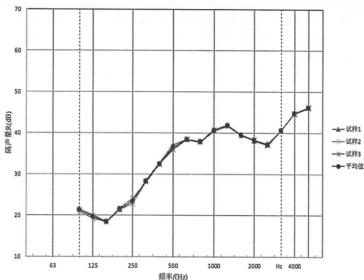
图 1 空气声隔声性能检测结果曲线图
