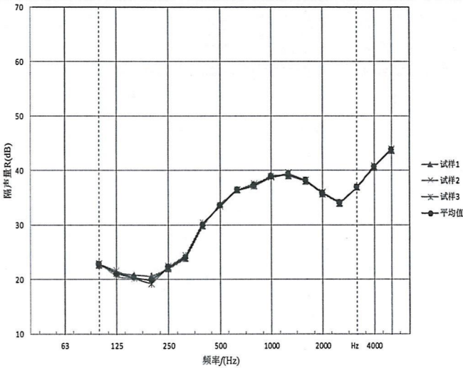
图 1 空气声隔声性能检测结果曲线图
