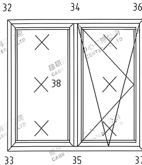
图1 试件热侧表面温度布点分布图
