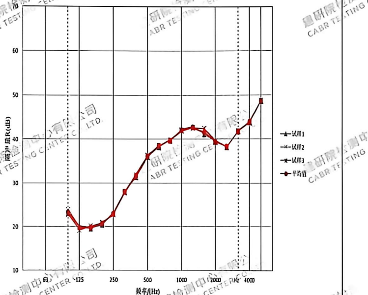
图 1 空气声隔声性能检测结果曲线图
