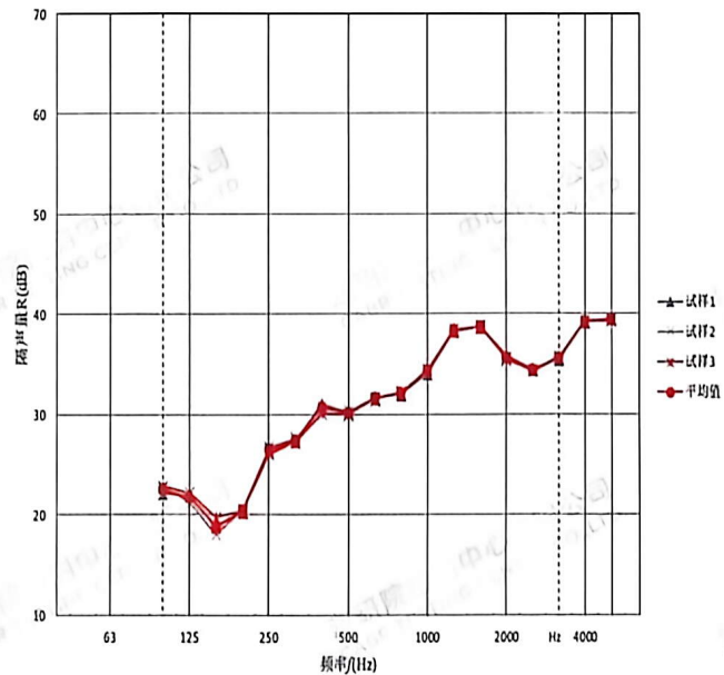
图 1 空气声隔声性能检测结果曲线图
