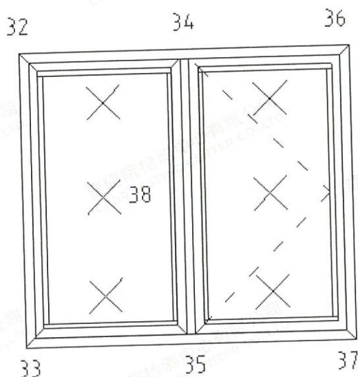
图1 试件热侧表面温度布点分布图
