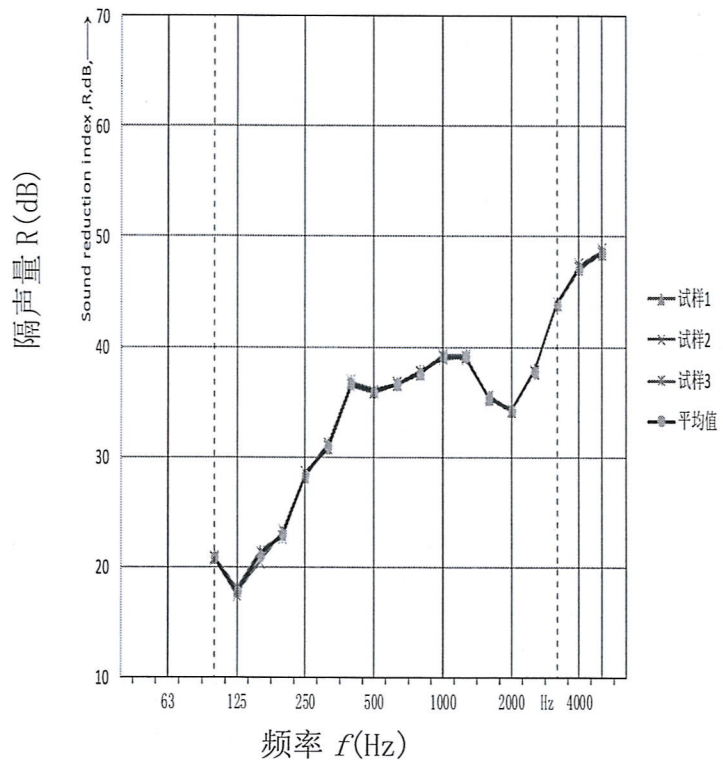
图 1 空气声隔声性能检测结果曲线图
