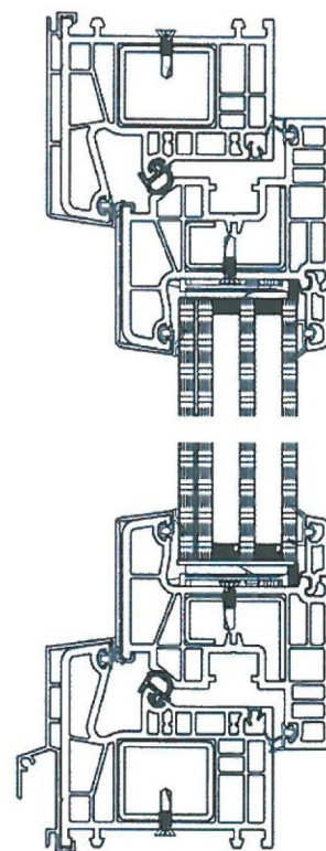
B — B
